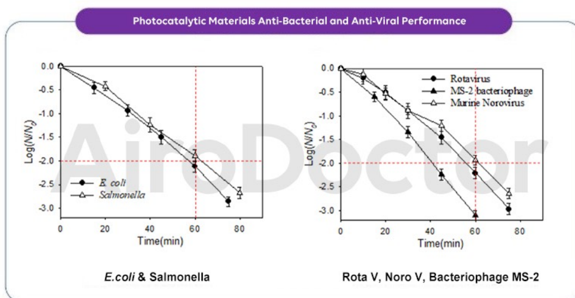
Fig. 2: Prestazioni antimicrobiche e antivirali del filtro fotocatalitico (1)
